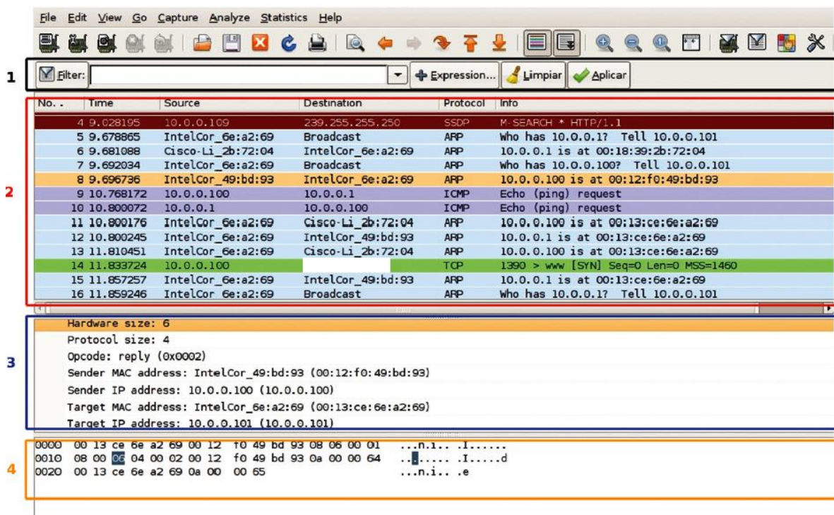
Figura 5- Áreas de Wireshark
