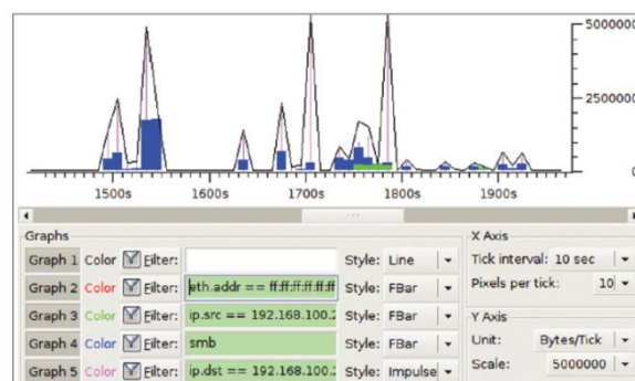
Figura 46- I/O Graph
