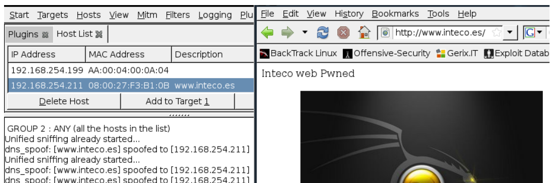
Figura 20- Ettercap
