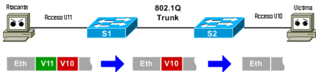
Figura 25- Vlan Hopping
