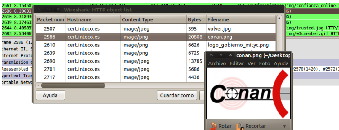
Figura 34- Objetos HTTP
